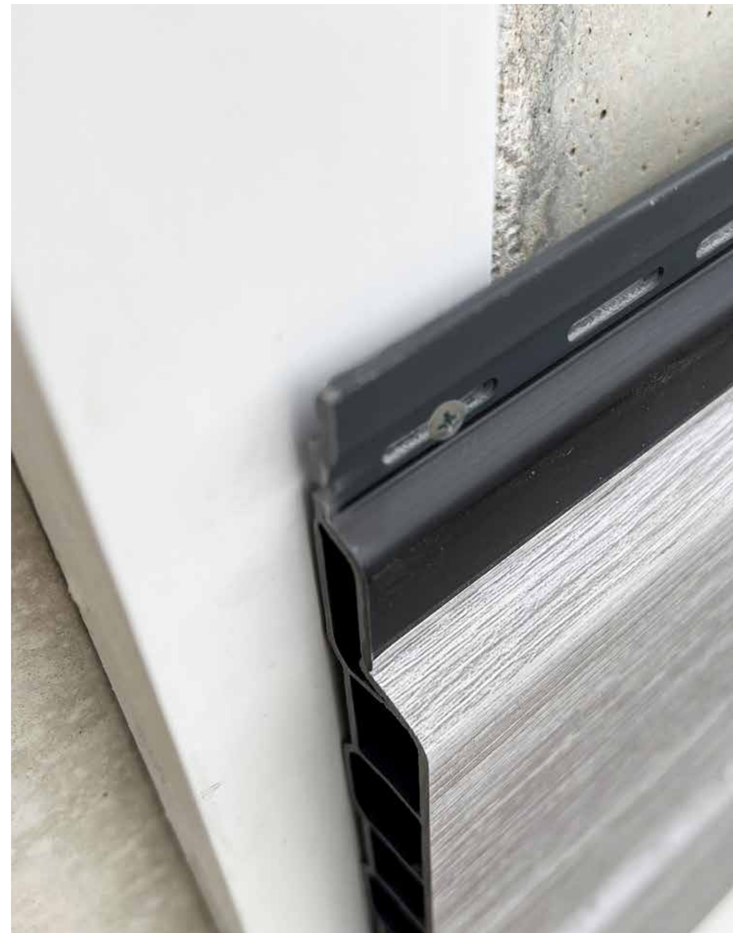
Dettaglio incastro pannello ISO15 montaggio a parete su distanziale ISO15 Panel Grout Line Detail with Wall Mounting on Spacer
