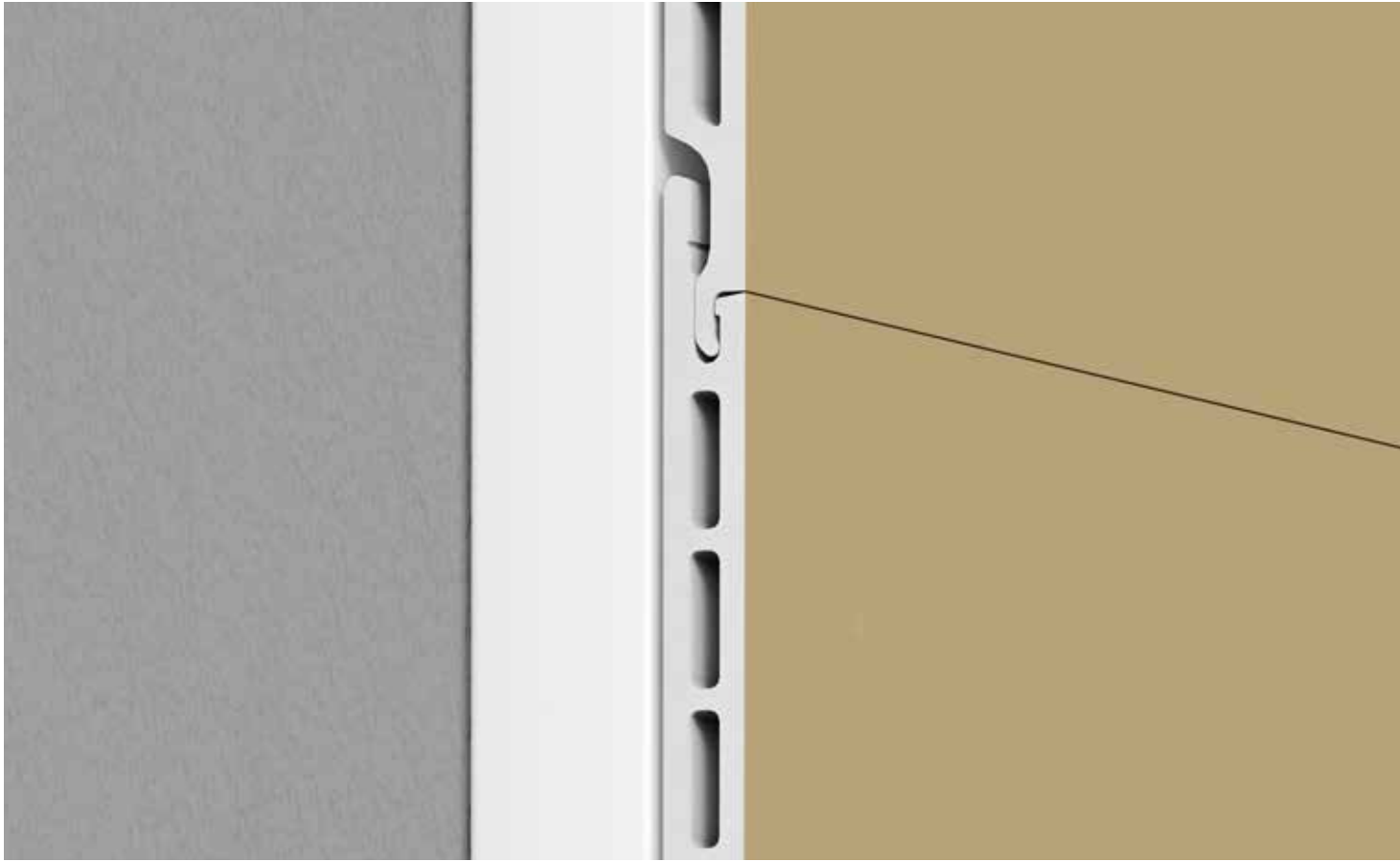
Dettaglio incastro pannello ISO33 montaggio a parete su distanziale ISO33 Panel Interlocking Details for Wall Mounting on Spacer
