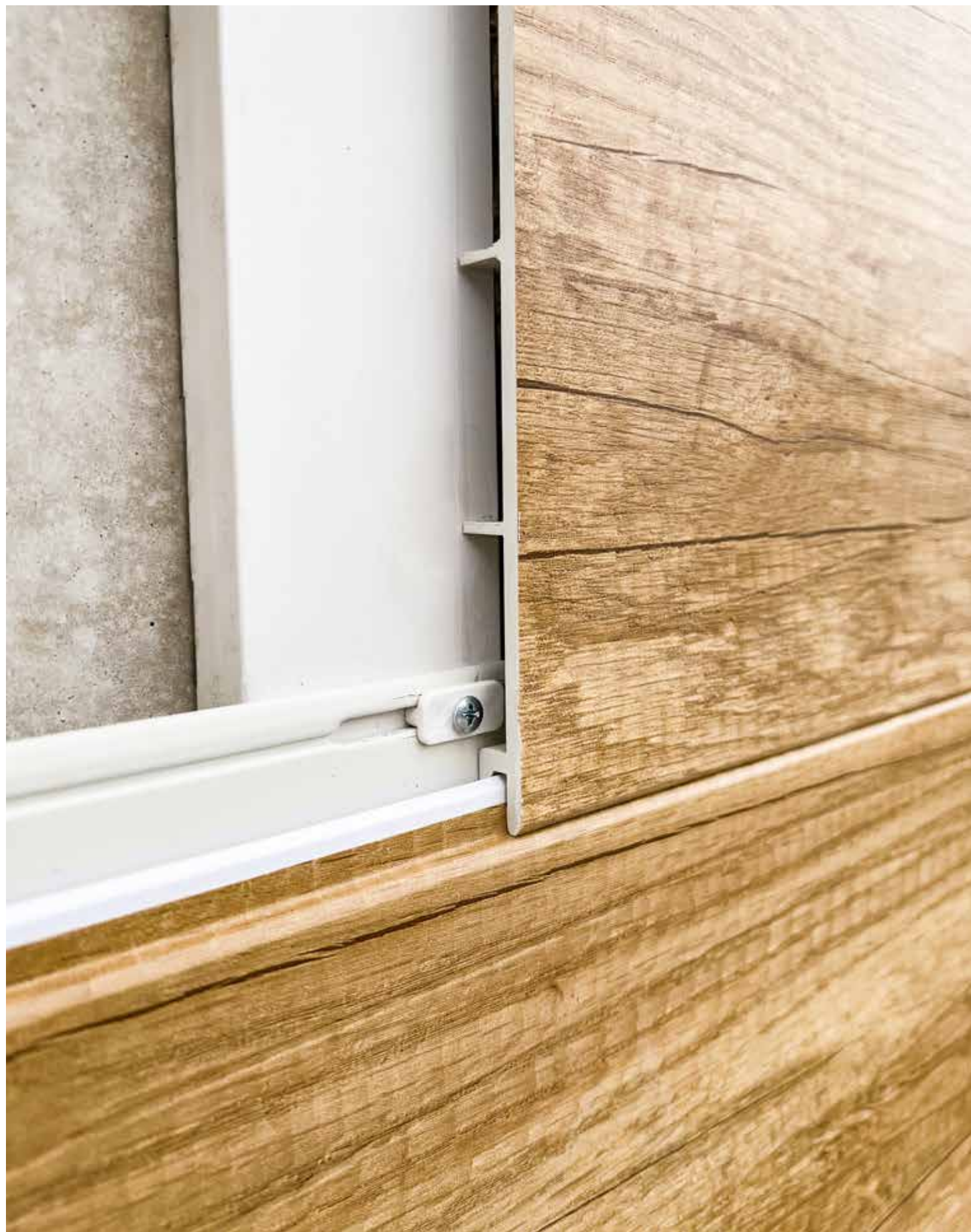
Dettaglio incastro pannello ISO20 con montaggio a parete su distanziale ISO20 Panel Interlocking Details with Wall Mounting on Spacer
