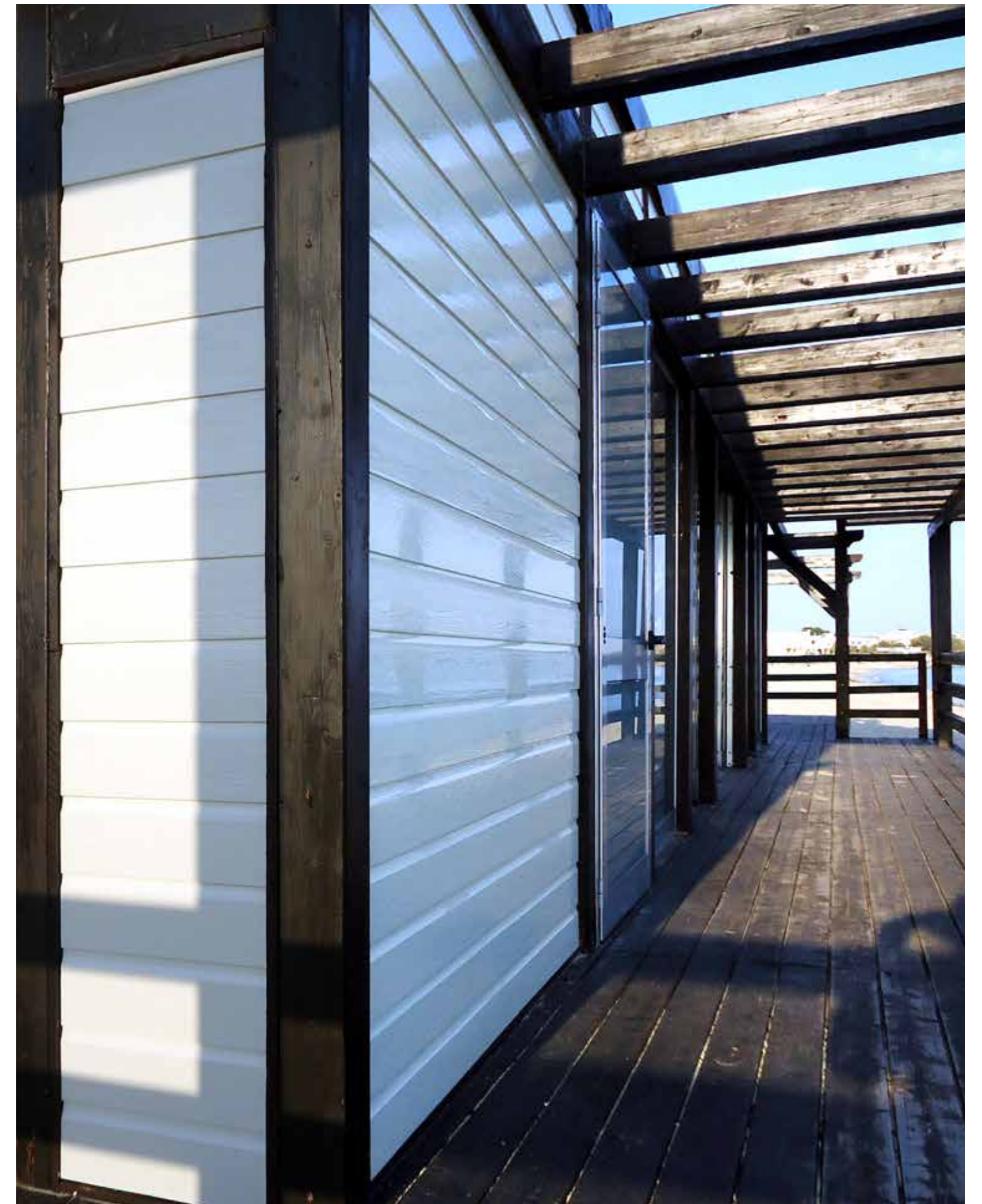
Installazione a Parete Orizzontale - ISOMUR - Legno Bianco Lucido Horizontal Wall Installation - ISOMUR - Glossy White Wood
