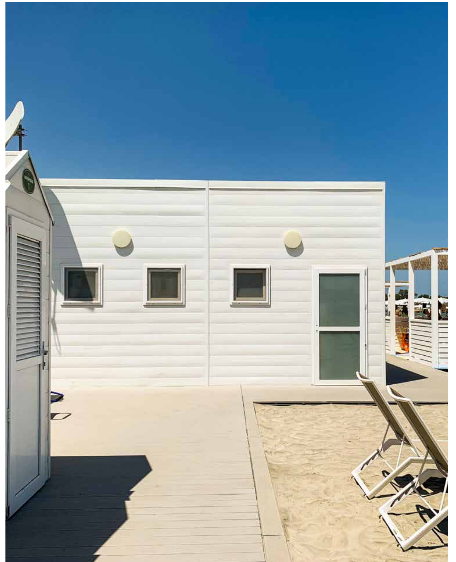
Installazione a Parete orizzontale - ISO20 - Legno Bianco Lucido
