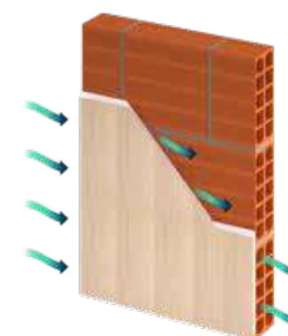
Ancoraggio diretto su parete priva di rivestimento di finitura Direct anchorage on wall without finish coating
